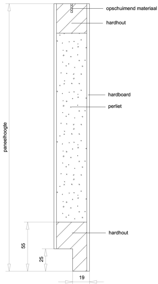
Doorsnede BB
