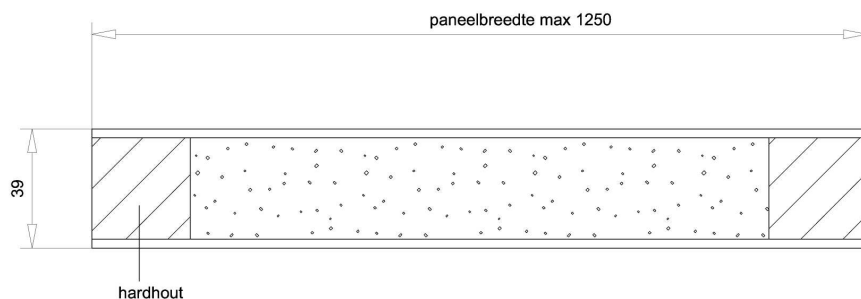
Doorsnede AA
