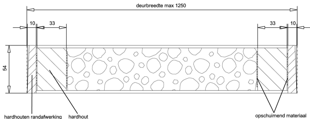
Doorsnede AA
