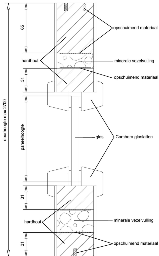
Doorsnede BB
