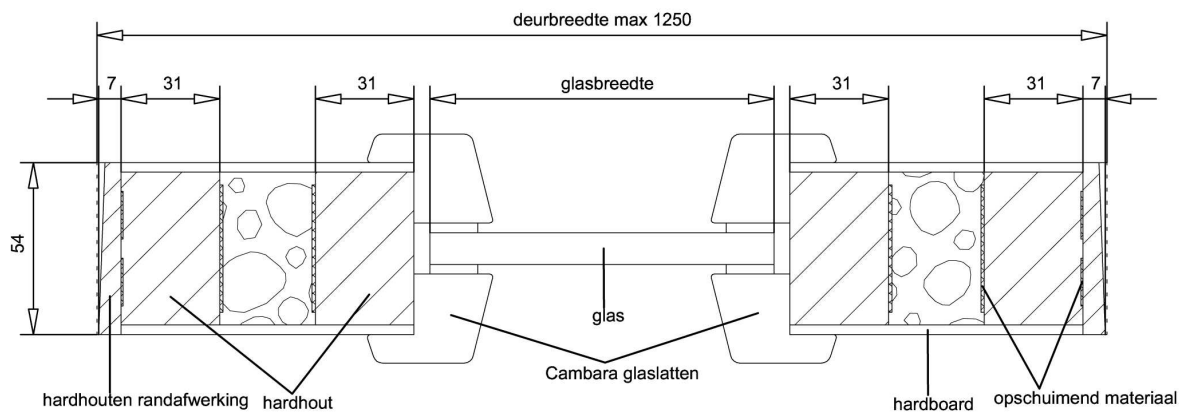
Doorsnede AA
