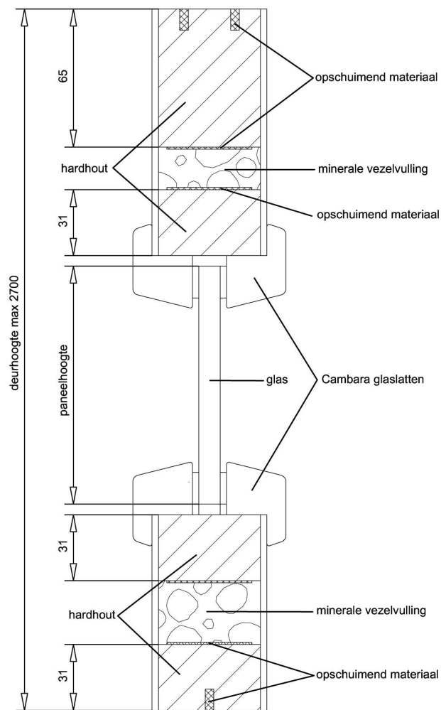
Doorsnede BB
