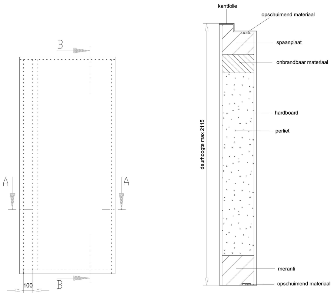
Doorsnede B-B
