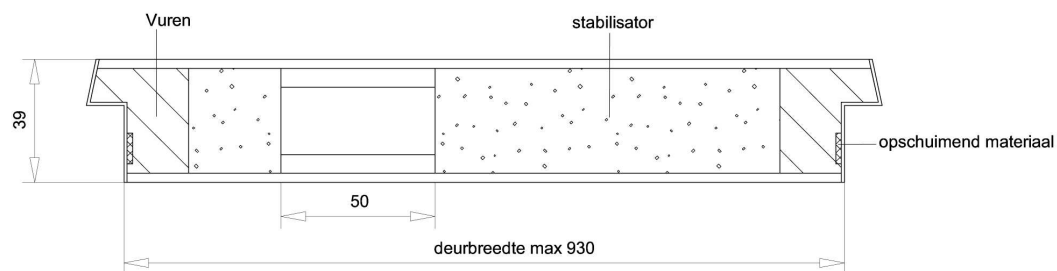
Doorsnede A-A
