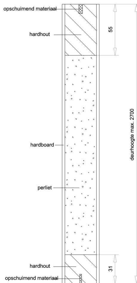
Doorsnede BB
