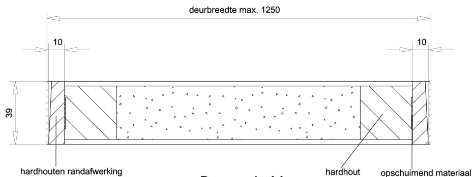
Doorsnede AA
