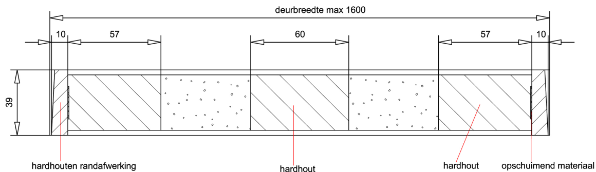
Doorsnede AA
