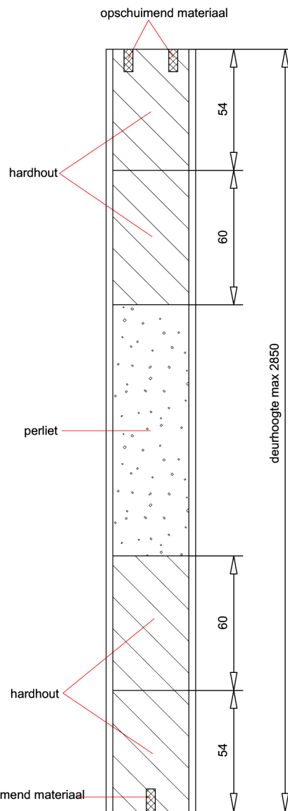
Doorsnede BB
