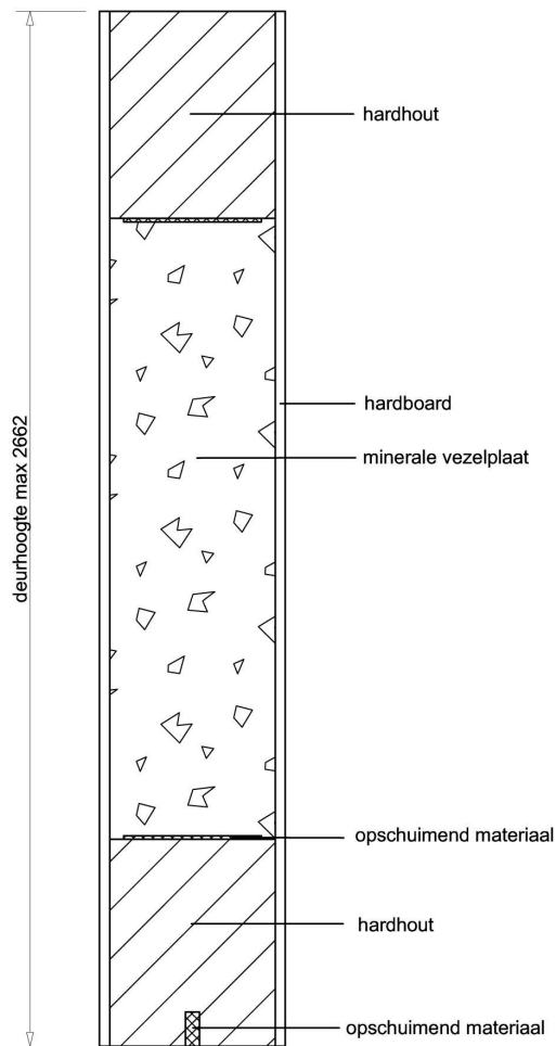
Doorsnede BB
