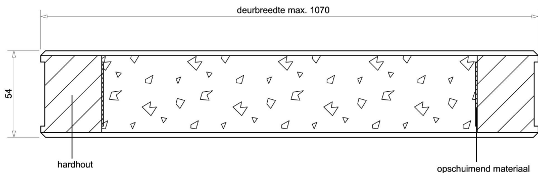
Doorsnede AA
