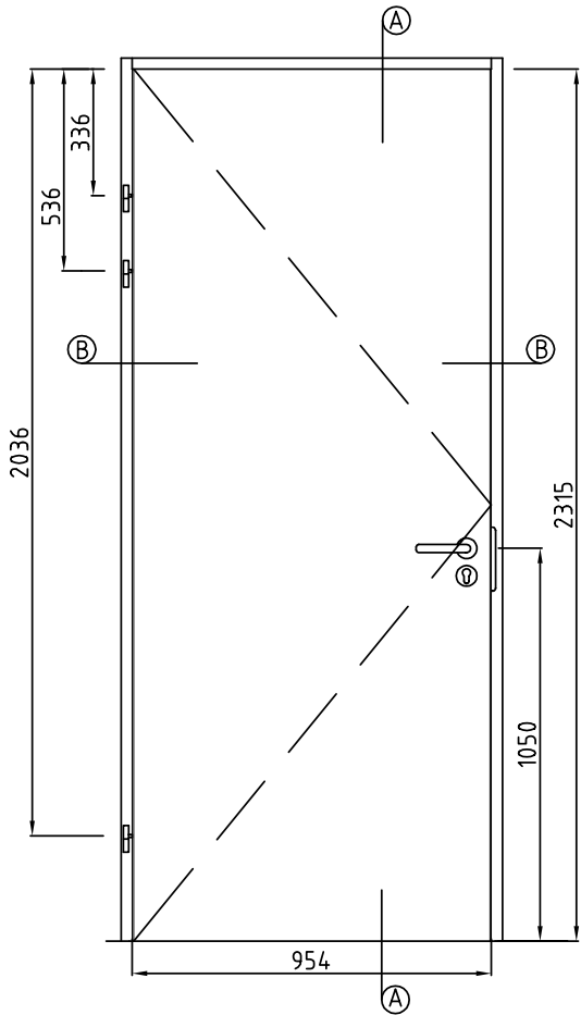
Vooraanzicht
