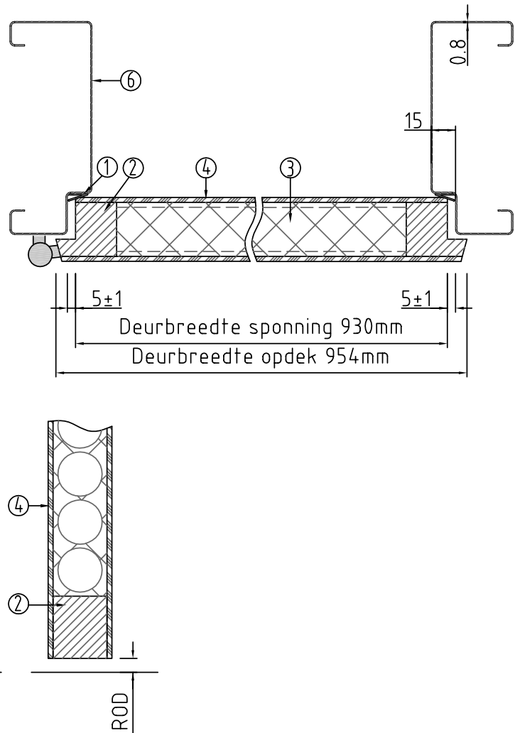
Doorsnede BB
